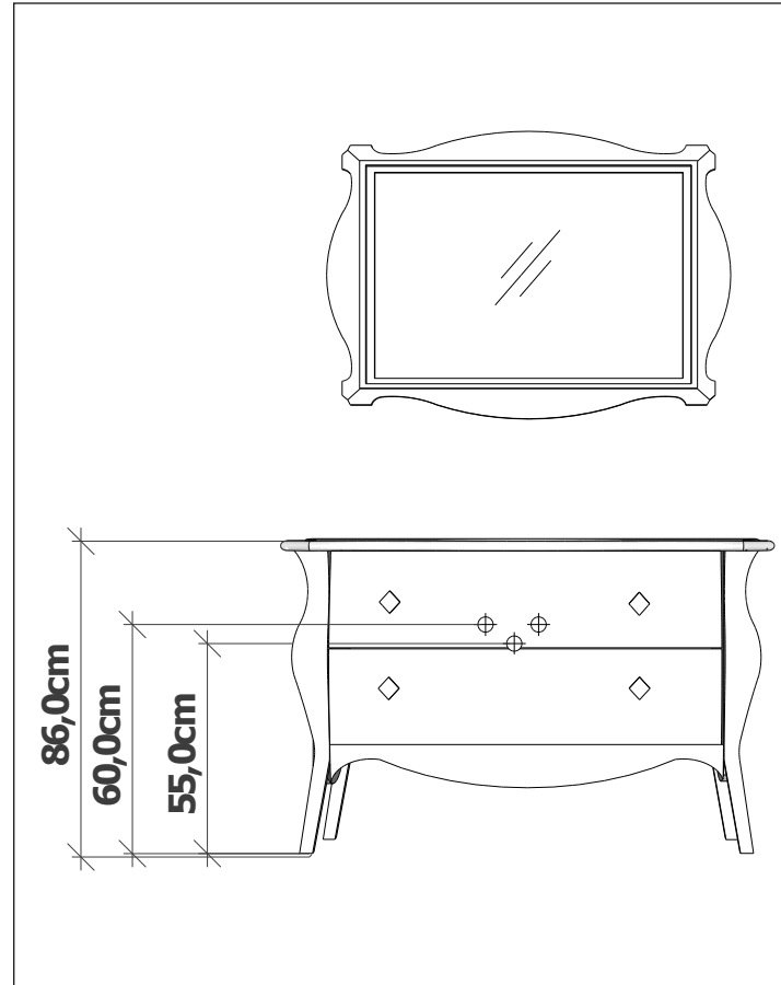
DIVERSO Su tesisatı ölçüsü Water installation dimension
