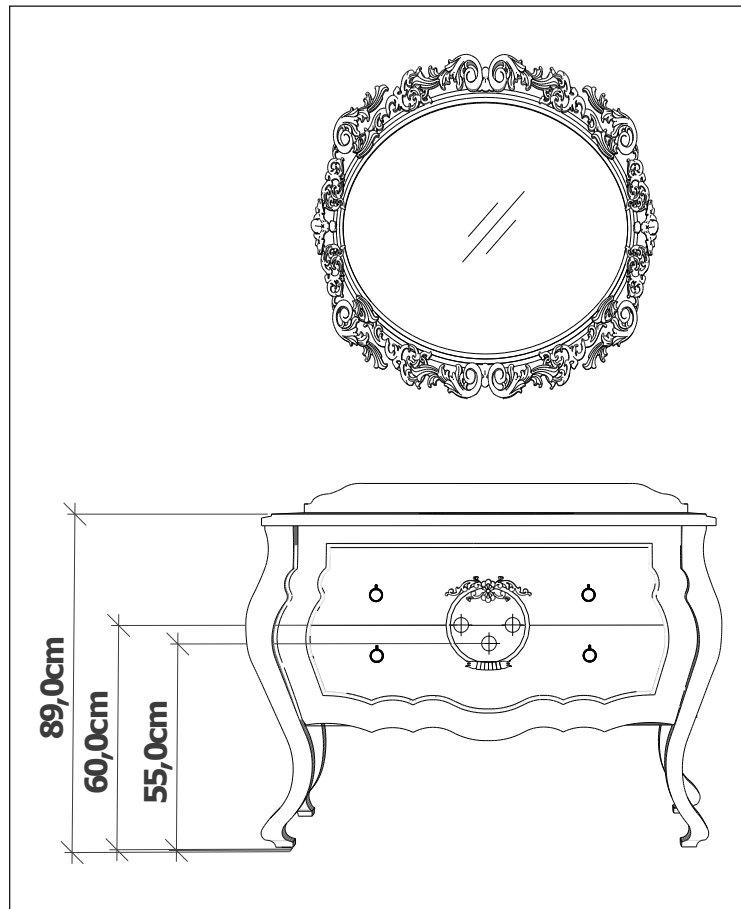
ORIENTE Su tesisatı ölçüsü Water installation dimension
