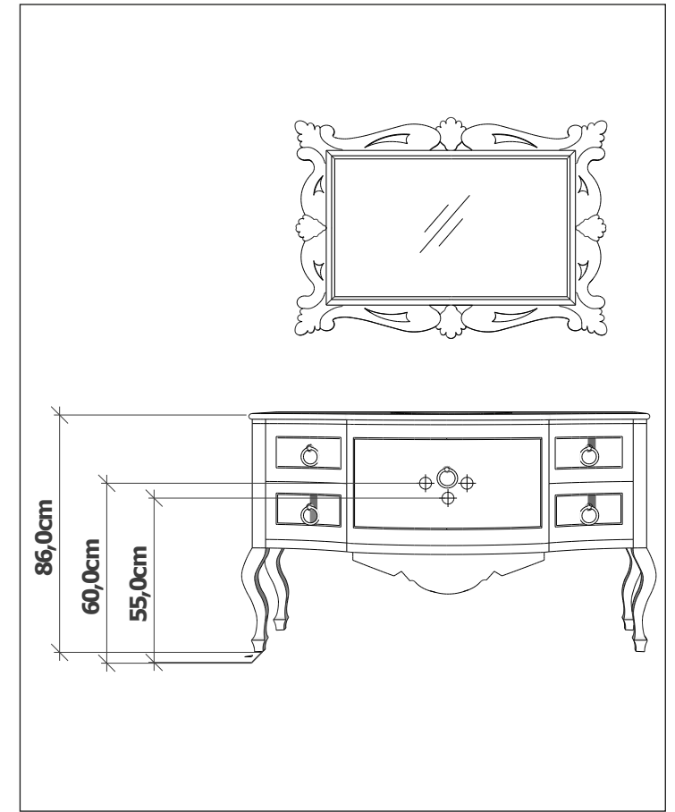
VICTORIA Su tesisatı ölçüsü Water installation dimension
