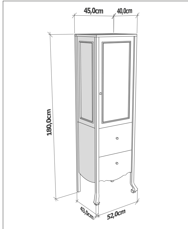
BERGAMO BOY DOLABI Tall cabinet
