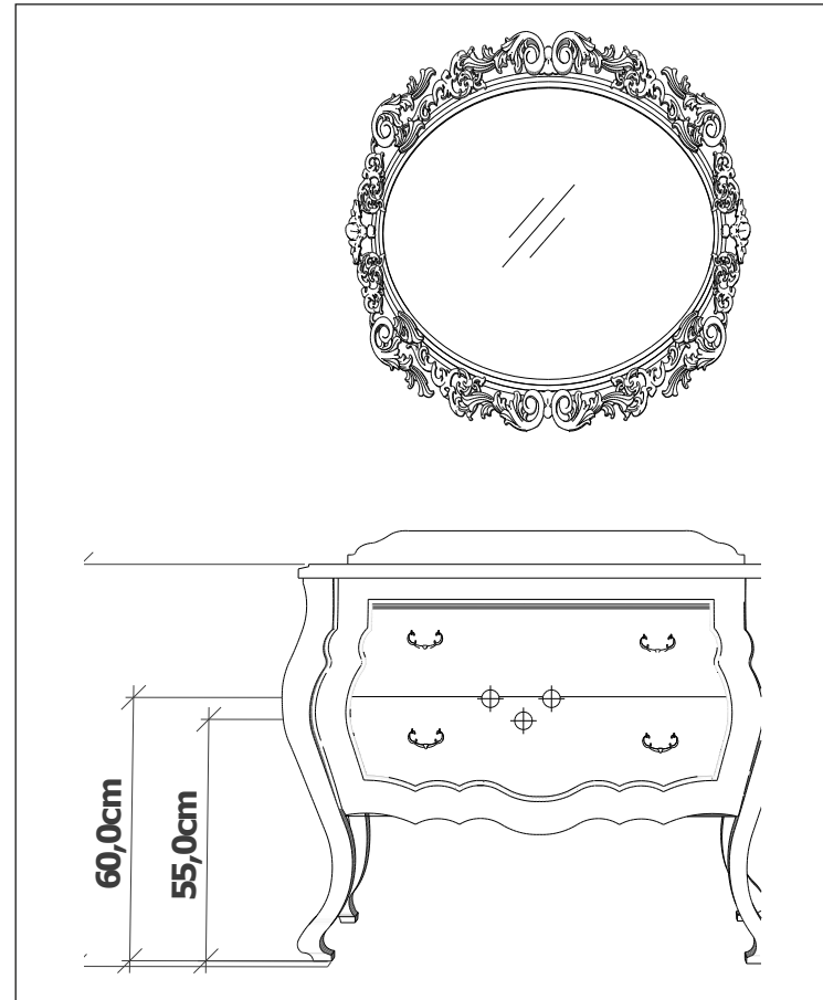
BERGAMO Su tesisatı ölçüsü Water installation dimension
