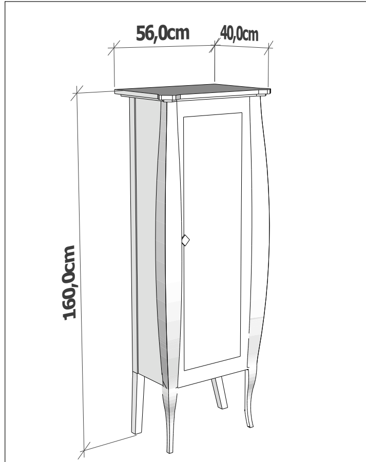
DIVERSO BOY DOLABI Tall cabinet
