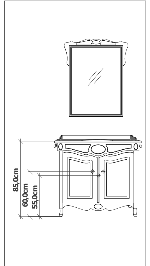
CLARA Su tesisatı ölçüsü Water installation dimension
