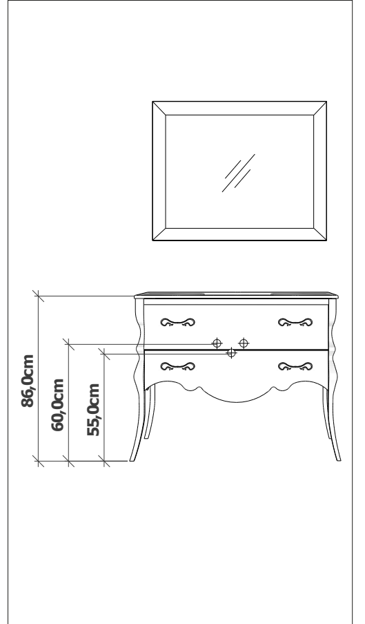
AMORE Su tesisatı ölçüsü Water installation dimension
