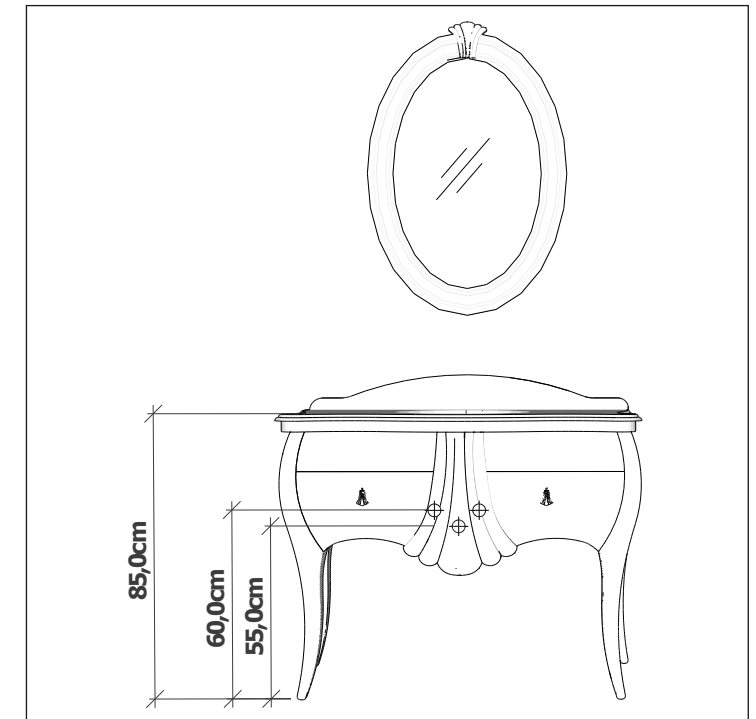
BALNOVO Su tesisatı ölçüsü Water installation dimension
