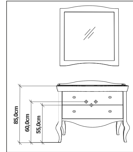
OLYMPIA Su tesisatı ölçüsü Water installation dimension
