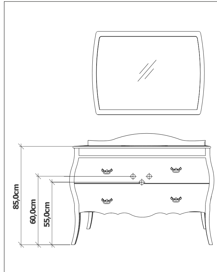
ARIA MINIMAL Su tesisatı ölçüsü Water installation dimension
