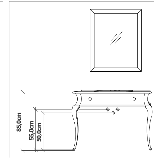
VIENNA Su tesisatı ölçüsü Water installation dimension
