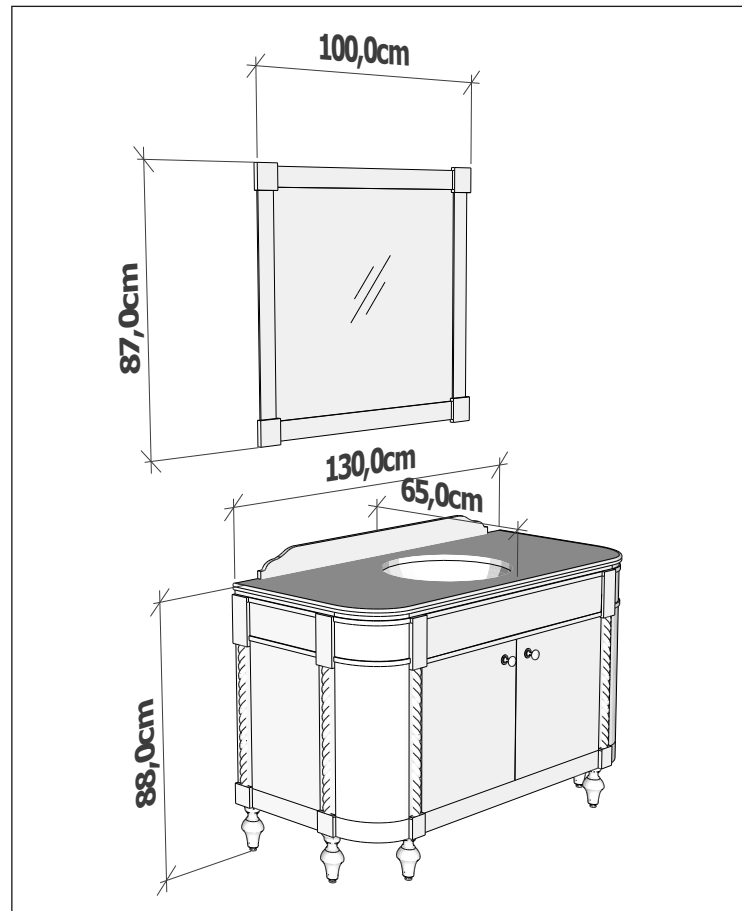
CLASSIC Su tesisatı ölçüsü Water installation dimension
